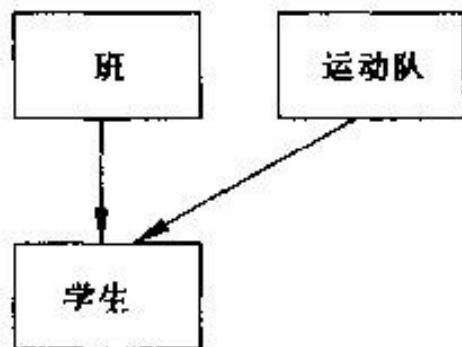
图 2-9 一个记录型有多个双亲
