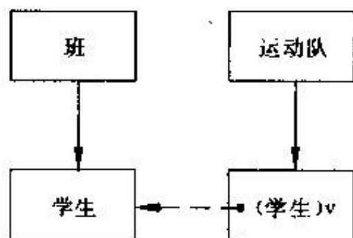
图 2-14 用虚拟记录表示的图 2-10 中的关系
