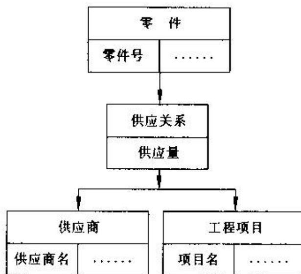
图 2-12 用 PCR 表示的图 2-11 的三元关系
