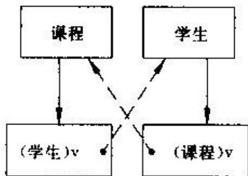
图 2-13 用虚拟记录表示 M:N 关系
